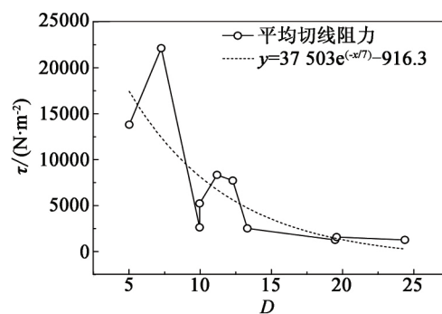
图 5 平均切线阻力随振动强度的变化
