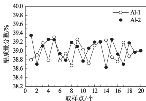
图 3 固含量 90% PBX 炸药中铝元素的质量分数
