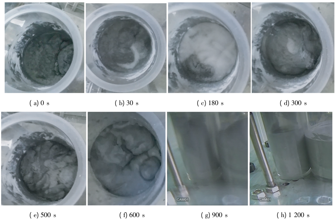
图 1 固含量 90% 的 PBX 炸药混合状态随时间的变化
