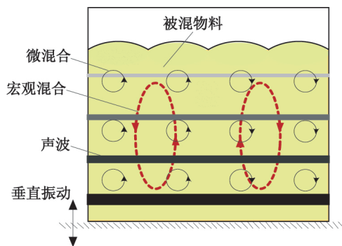
图 4 共振声混合机理示意图
